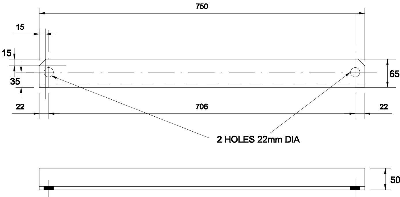
ITEM 2 65 x 50 x 8 ANGLE - 750 LONG
