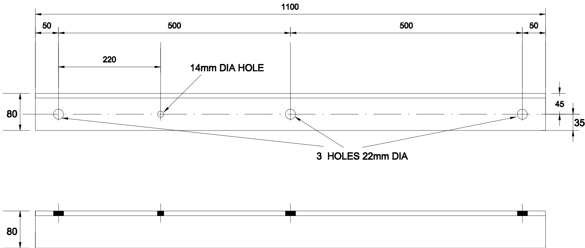
ITEM 1 80 x 80 x 10 ANGLE - 1100 LONG
